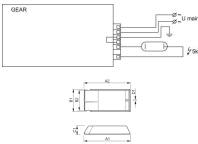
Technische Daten Philips HID-PV C 35 / I CDM 220-240V 50/60Hz für 35W
